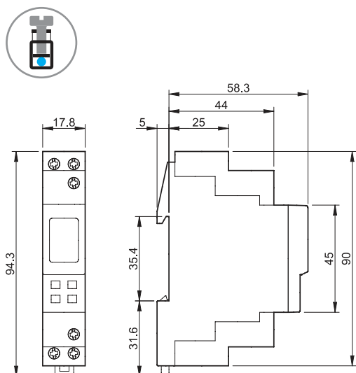
12.71 Schraubklemmen
