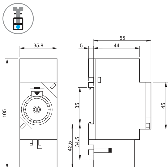
12.31 Schraubklemmen
