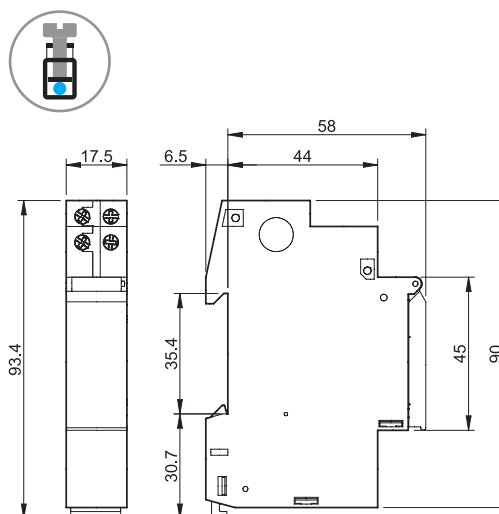
12.11 Schraubklemmen
