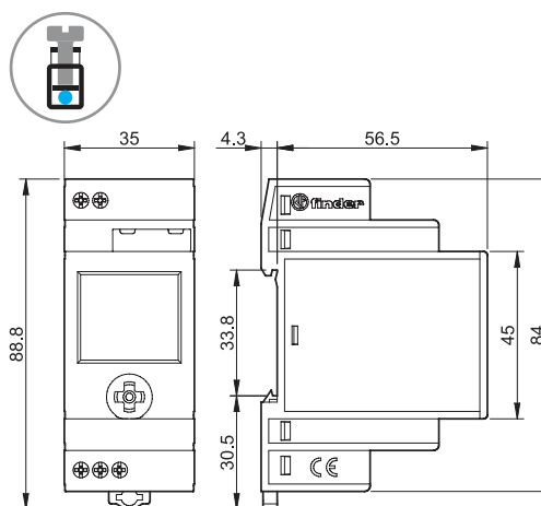
12.51/12.81 Schraubklemmen
