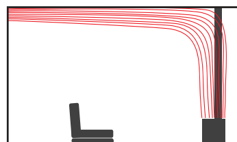
WÄRMEVERTEILUNG OHNE OFEN VENTILATOR
