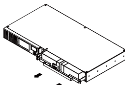
5. Zainstaluj nowe akumulatory. Podłącz akumulatory, zamontuj osłonę oraz panel czolowy, postępując zgodnie z instrukcją powyżej w odwrotnej kolejności. Ładuj akumulatory co najmniej
