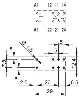
Ansicht auf die Anschlüsse 5.3 mm Pinlänge für Leiterplatte oder Fassung Serie 95
