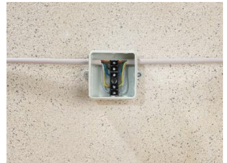
2. Verlegung und Verdrahtung der Kabel. Anschließend Abzweigkasten bis auf das Einfüllloch schließen!
