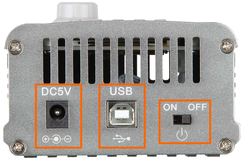
Anschluss USB-Interface Ein-/Ausschalter Spannungsversorgung 5V DC
