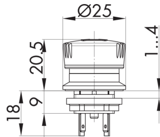
Maßskizze:
