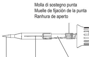
Punta Punta de soldar Ponta de solda Fessura di serraggio Ranura Elemento riscaldante Resistencia Elemento térmico
