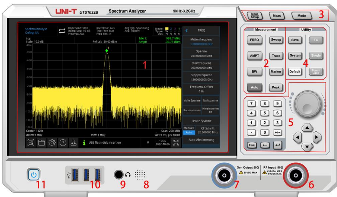
Abbildung 1-1 Frontplatte
