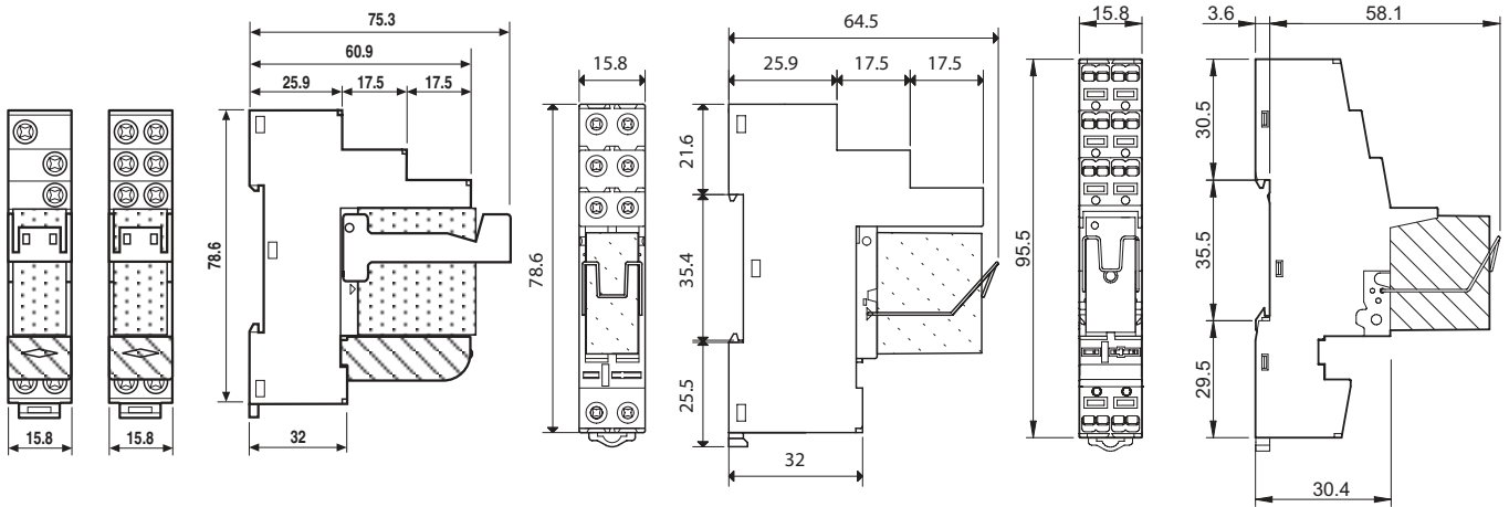
Typ 48.31 / 48.32 / 48.52 / 48.61 / 48.62 Schraubklemmen
