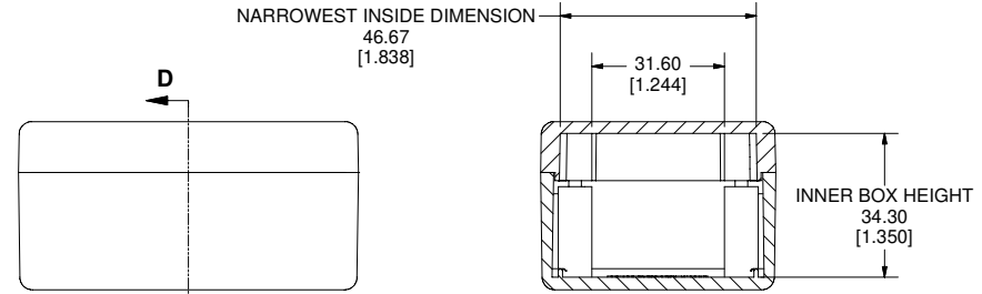
SECTION D-D SCALE 1 : 1
