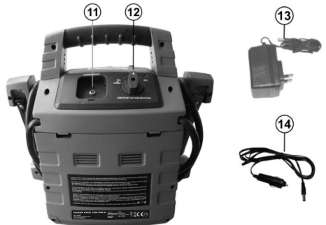
Bild 2: Übersicht, Rückseite
