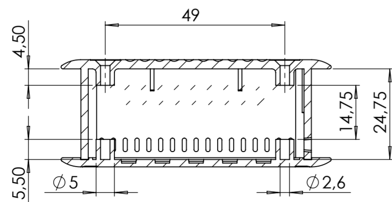
SEZIONE A-A
