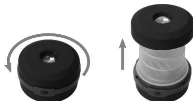
Figure 4 : Déploiement du corps transparent
