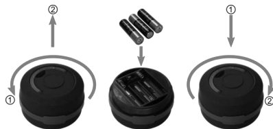
Bild 3: Batterie einsetzen
