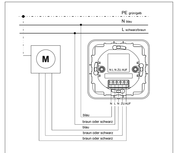
Abb1. Anschlusskizze Art.320050
