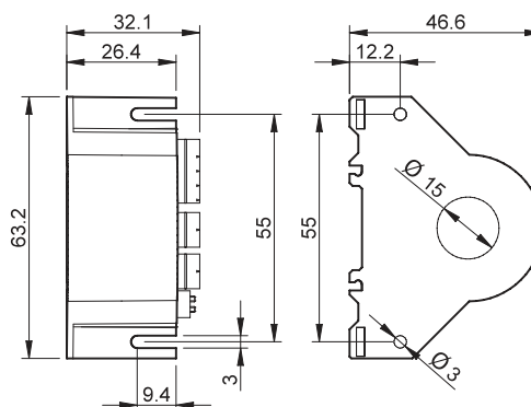
Typ 6M.BU
