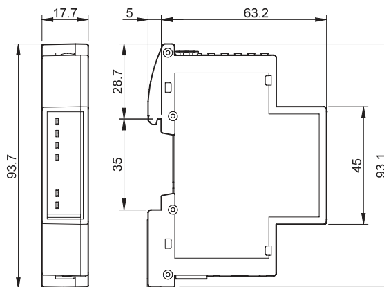
Typ 6M.BU
