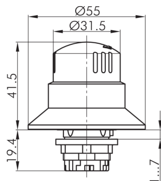
Maßskizze:
