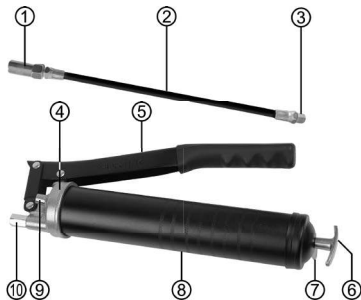
Figura 1 : Schema
