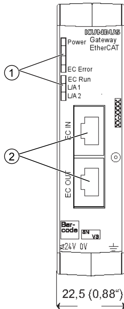
Abb. 2: Frontansicht
