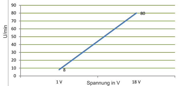
G298-12V
