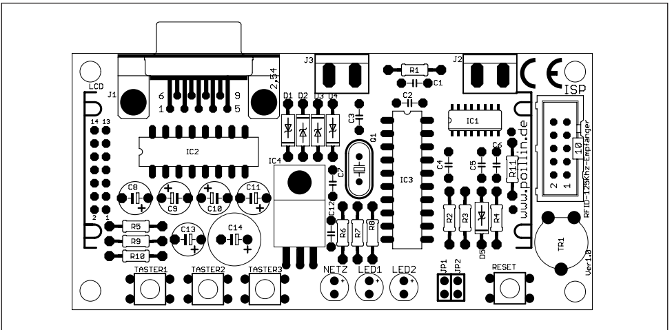
Bestückungsplan
