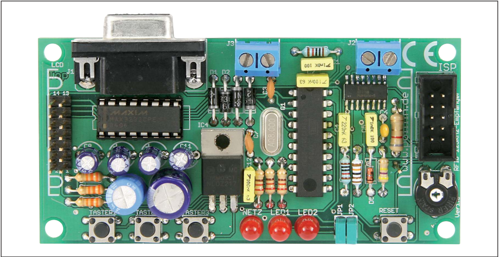
RFID-125kHz-Empfänger-Bausatz
