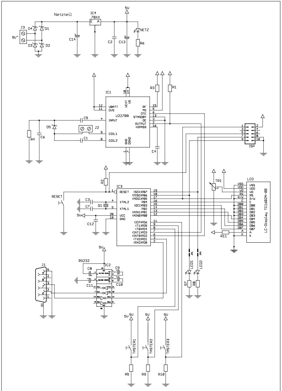
Schaltplan für den RFID-125kHz-Empfänger-Bausatz
